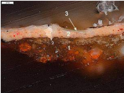
SPA-2, 200 X
